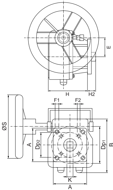
Quadro lato attuatore / Actuator Square
